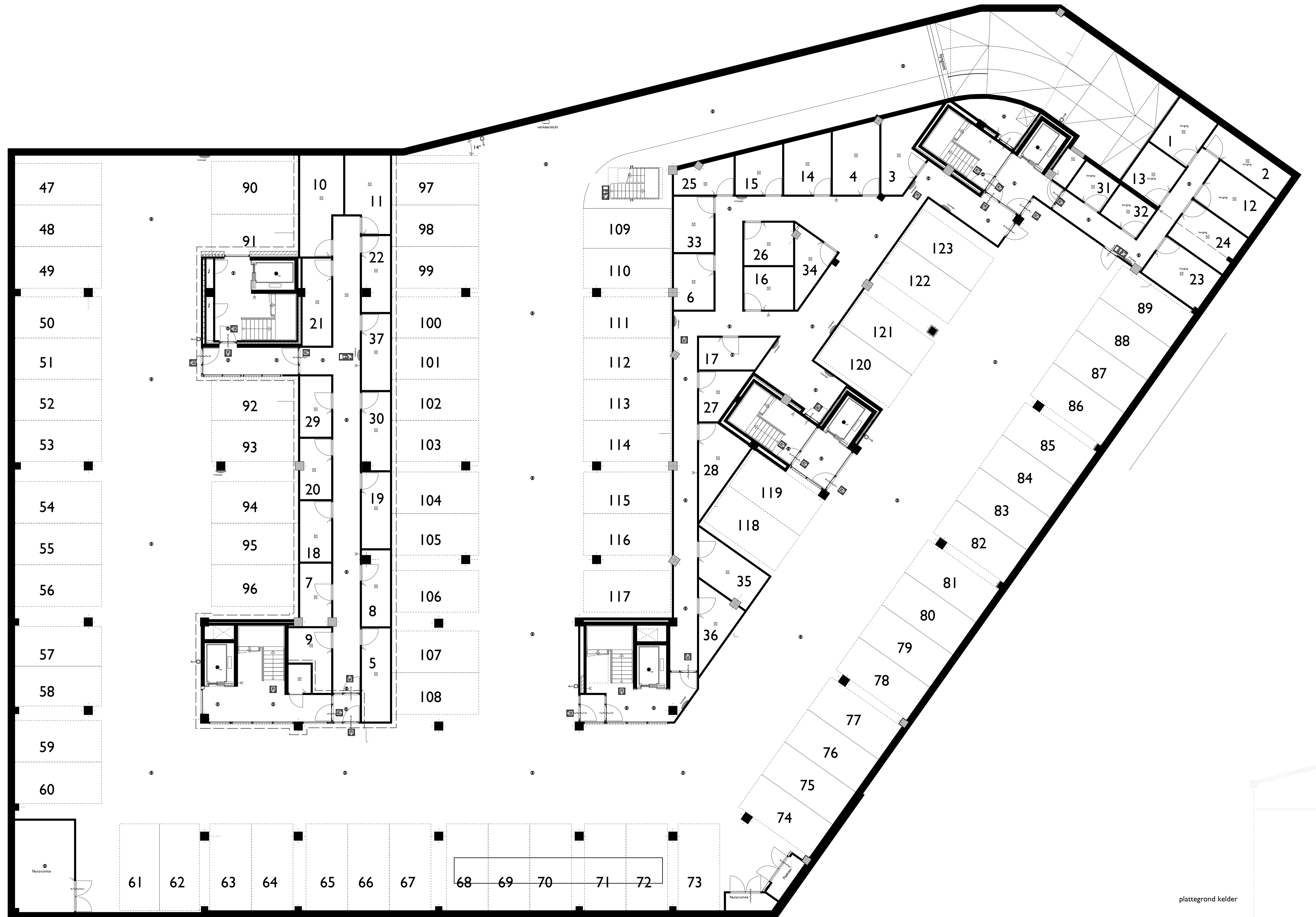
plattegrond kelder
